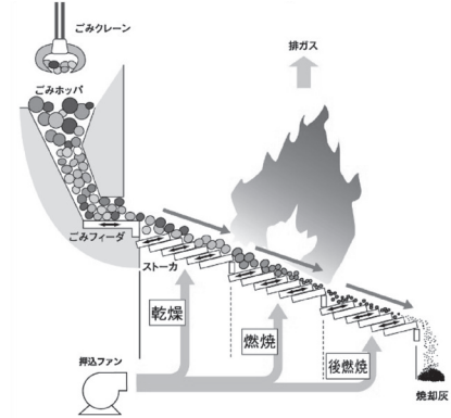
※ストーカ式ごみ焼却炉のしくみ
